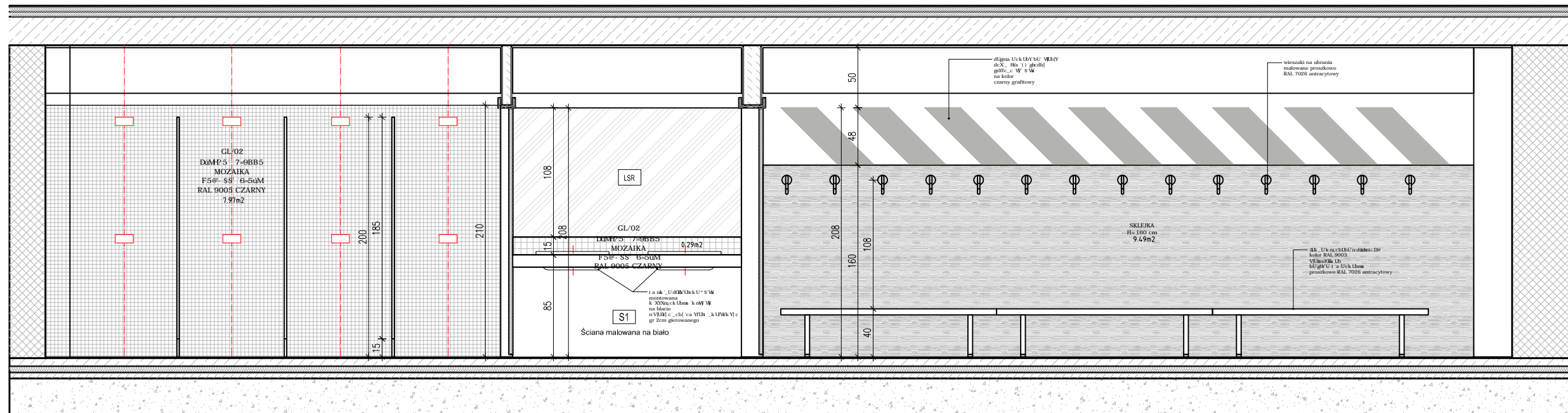
WIDOK A-A
