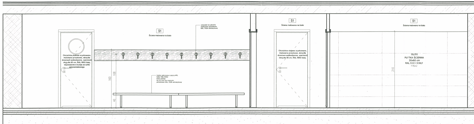
WIDOK B-B
